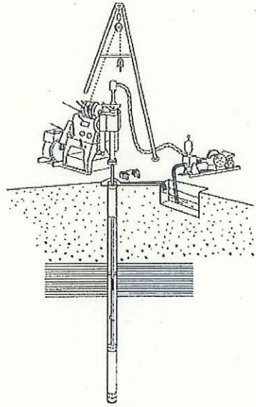
【図3 ボーリング調査（出典：国土交通省四国地方整備局松山河川国道事務所ホームページ）】
