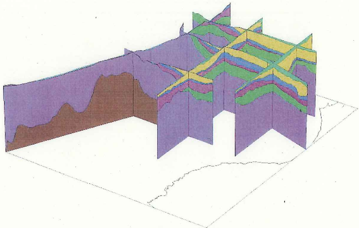
地質断面のパネルダイヤグラム
