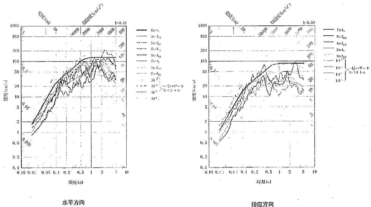
【図2-4 一様ハザードスペクトルと基準地震動 S_{s-1} ～ S_{s-5} の比較の例（出典：第402回原子力発電所の新規制基準適合性に係る審査会合・資料2-4「玄海原子力発電所地震について」・376ページ】
