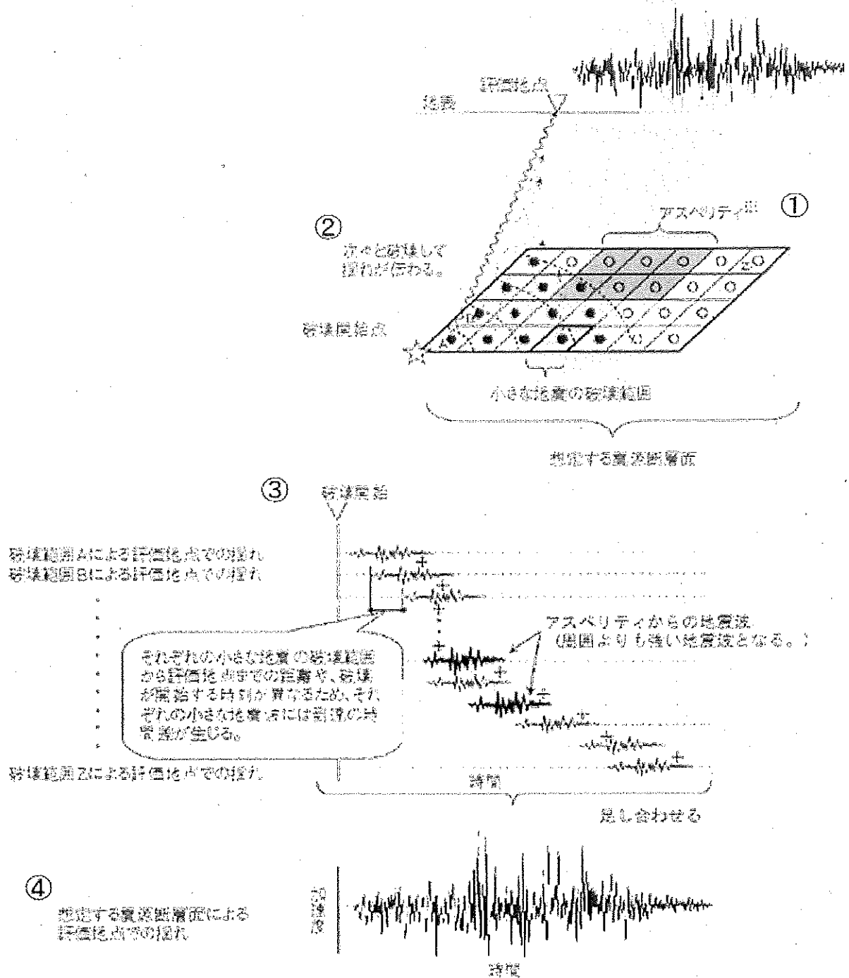
【図19 断層モデルの手法の概念について（出典：原子力安全委員会資料に一部加筆）】
