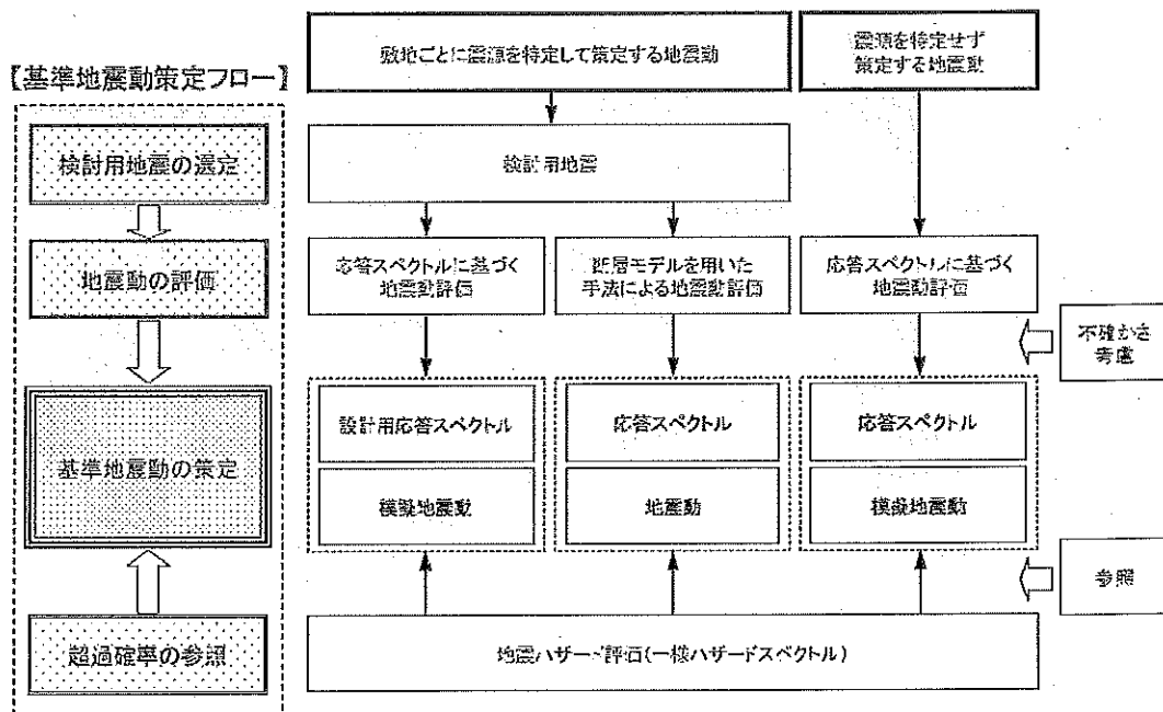
【図 2 2 基準地震動の策定に係る審査フロー（出典：地震動審査ガイド）】
