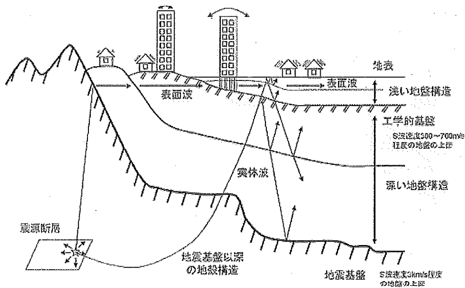
【図15 地下構造モデルの模式図（出典：強震動予測レシポ・乙第99号証）〔乙第79号証の改訂版〕】
