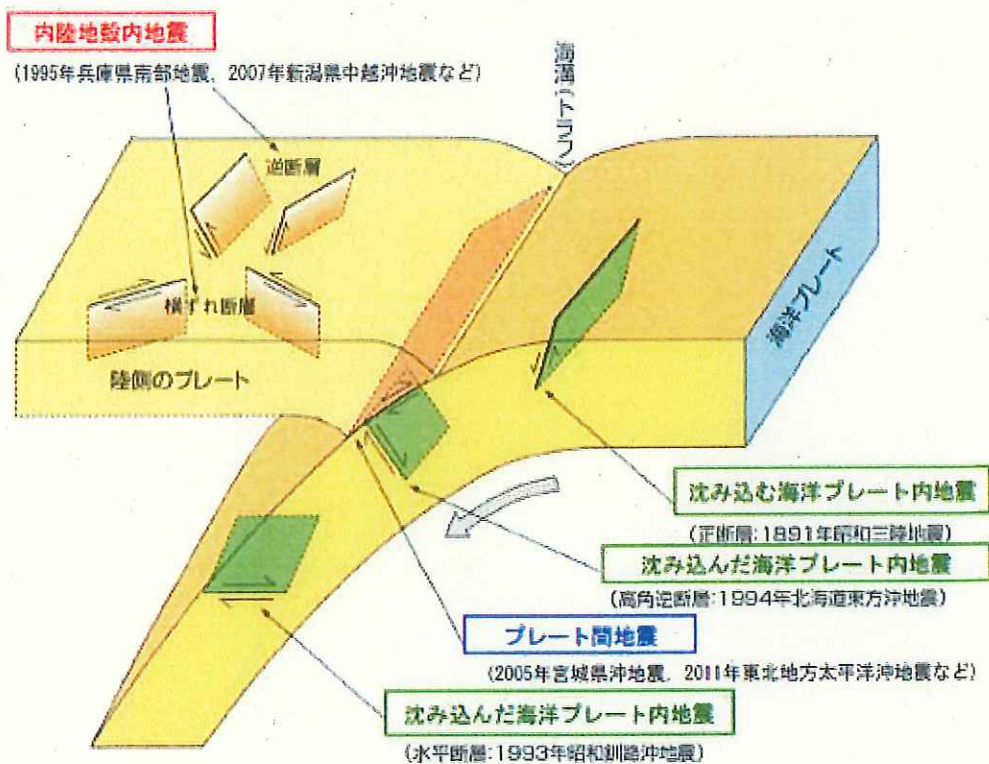
【図10 地震の発生様式（出典：原子力安全・保安院監修，独立行政法人原子力安全基盤機構編集・発行「原子力発電所の耐震安全性」（平成19年7月）に加筆）】
