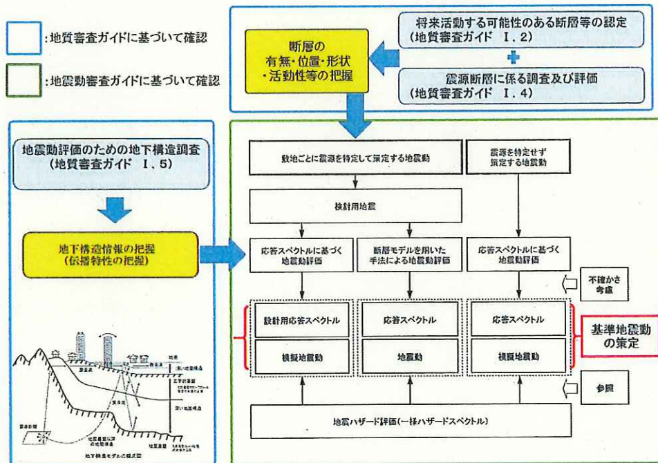
【図1 基準地震動策定フローと地質審査ガイド・地震動審査ガイドの役割（出典：地震動審査ガイドの図-1・1ページと強震動予測レシピ（乙第99号証）〔乙第79号証の改訂版〕23ページの図に加筆して作成。）】
