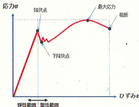
【図16 弾性範囲と塑性範囲】
